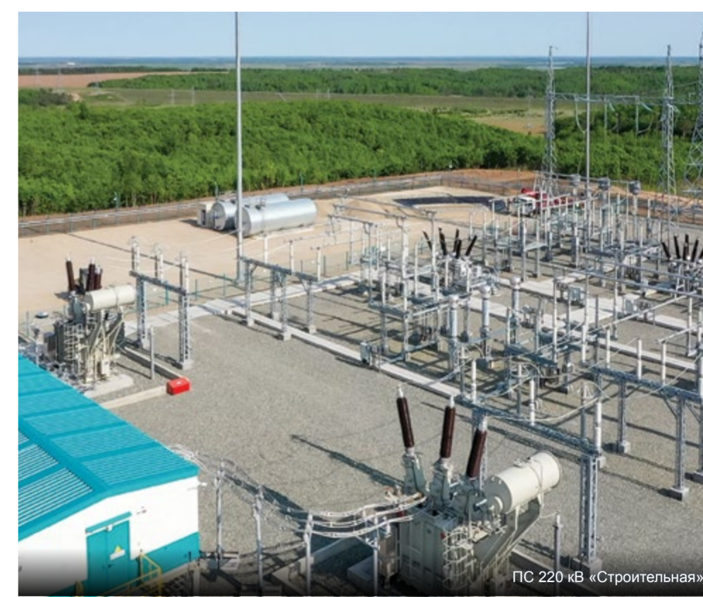
ПС 220 кВ «Строительная»
